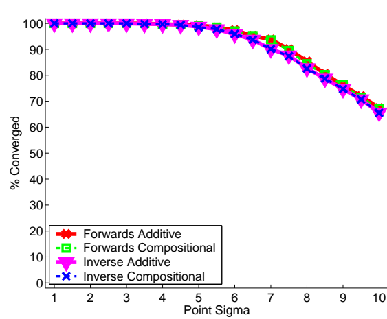
(d) Frequency of Convergence for “Knee” image
